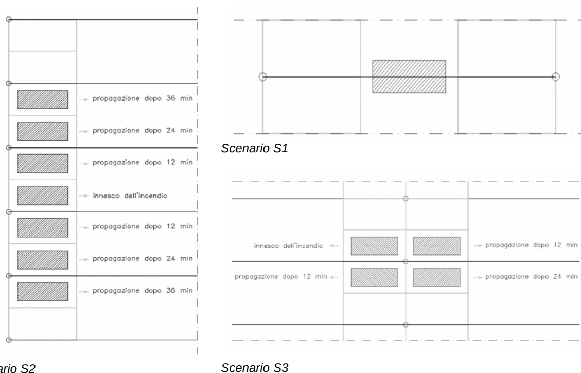
Illustrazione V.6-1: Schematizzazione degli scenari di incendio di progetto
